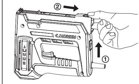
Fig. 3 Trek de pusherassemblage uit
