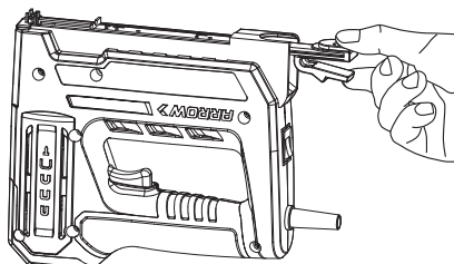
Figure.3 Tirez sur l'ensemble poussoir
