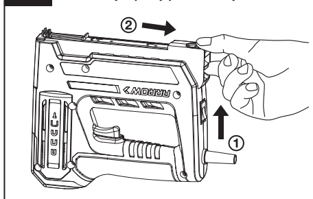
Slika 2 Hitro snemljiv spodnji polnilni nabojnik
