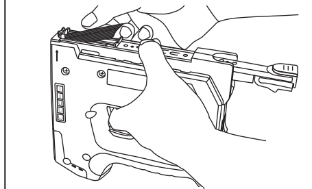
Fig. 5 Leg spijkers aan de linkerkant van het kanaal met punten naar boven
