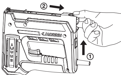
Fig. 2 Caricatore a Sgancio Rapido dal Basso
