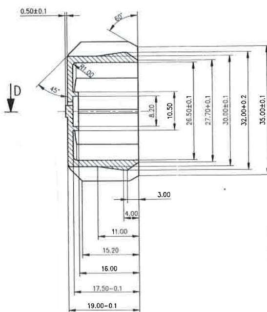
Schnitt C-D
