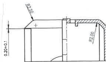
Schnitt C-D
