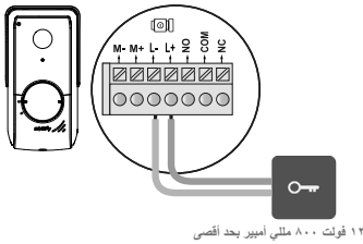
١٢ فولت ٨٠٠ مللي أمبير بحد أقصى
