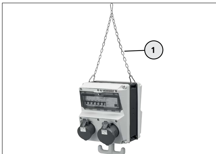
Combinazione di prese di corrente come quadro di distribuzione sospeso
