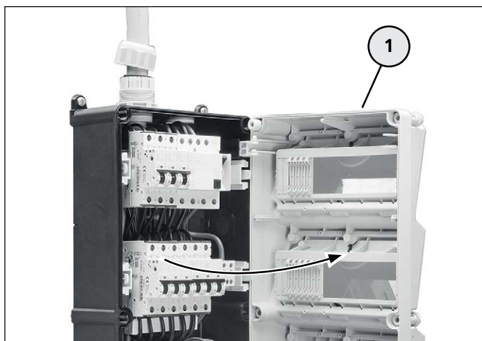
Gerät öffnen
