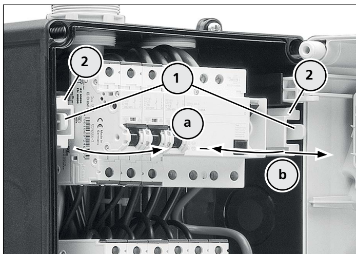
Estrarre le rotaie portanti
