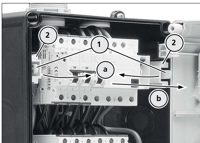
Tragschienen herausziehen
