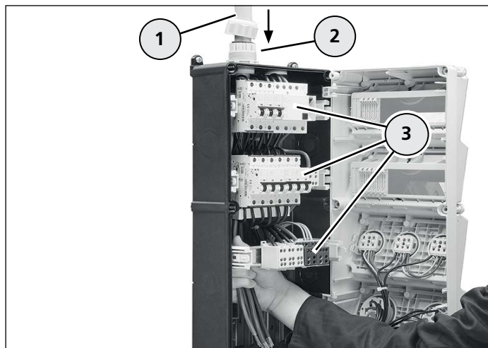
Apparaat aansluiten
