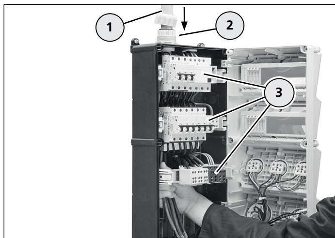
Gerät anschließen
