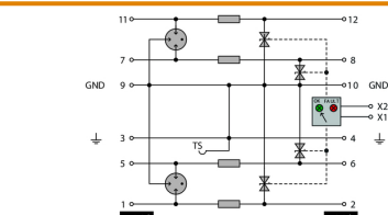
Komplettmodul direkte Erdung, mit Fernmeldung
