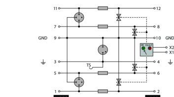
Komplettmodul indirekte Erdung, mit Fernmeldung Komplettmodul
