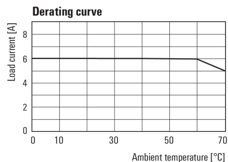
DC terheléskorlátozási görbe
