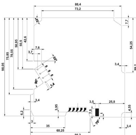
A NYÁK sorkapocs csatlakozású (MKDSO) ME MAX U-U1 NYÁK lap méretrajza, nézet a beültetési oldalról
