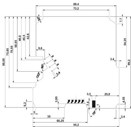
A dugaszolható csatlakozású (MSTBO) ME MAX U-U1 NYÁK lap méretrajza, nézet a beültetési oldalról
