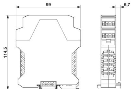
A kéteemeletes felső résszel rendelkező ME...TBUS... elektronikához méretei
