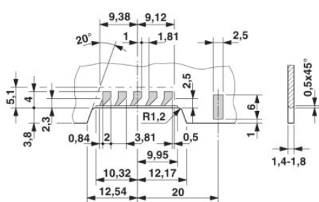
Az ME.../TBUS... NYÁK lap méreteiraja a kételeetes felső rész alkalmazása esetén
