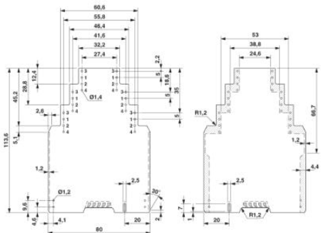
Az ME.../TBUS... NYÁK lap méreteiraja a háromemeletes felső rész alkalmazása esetén
