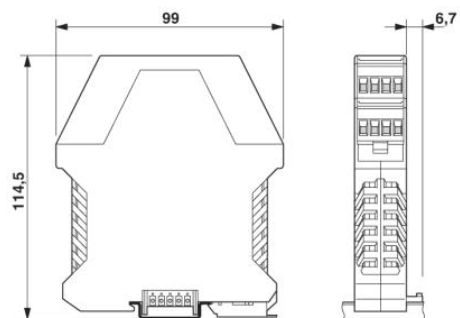
A kéteemeletes felső résszel rendelkező ME...TBUS... elektronikához méretei
