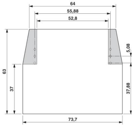
Sematikus rajz
