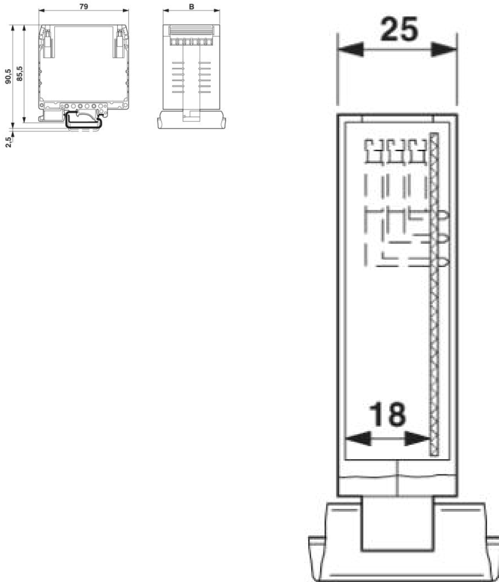
UEGM 25... és UEGM 27,5-SMD 1 NYÁK lappal, 6 pólusú ill. 12 pólusú (FS/FS)
