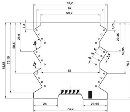
A NYÁK sorkapocs csatlakozású (MKDSO) ME MAX ...F 3-3 NYÁK lap méretrajza, nézet a beültetési oldalról
