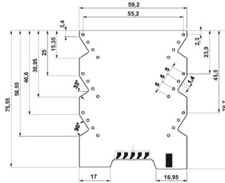
A dugaszolható csatlakozású (MSTBO) ME MAX ...SF 3-3 NYÁK lap méretrajza, nézet a beültetési oldalról
