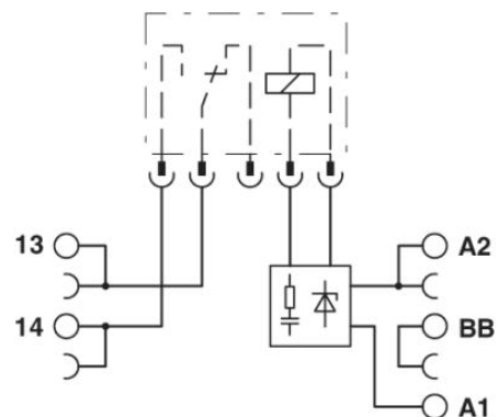
DC kimenet
