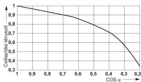
Élettartam-csökkenési tényező különböző cos phi értékeknél
