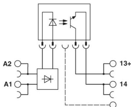
Kapcsolási rajz
