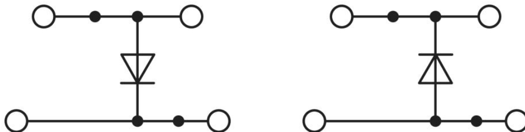
Kapcsolási rajz
