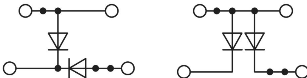
Kapcsolási rajz
