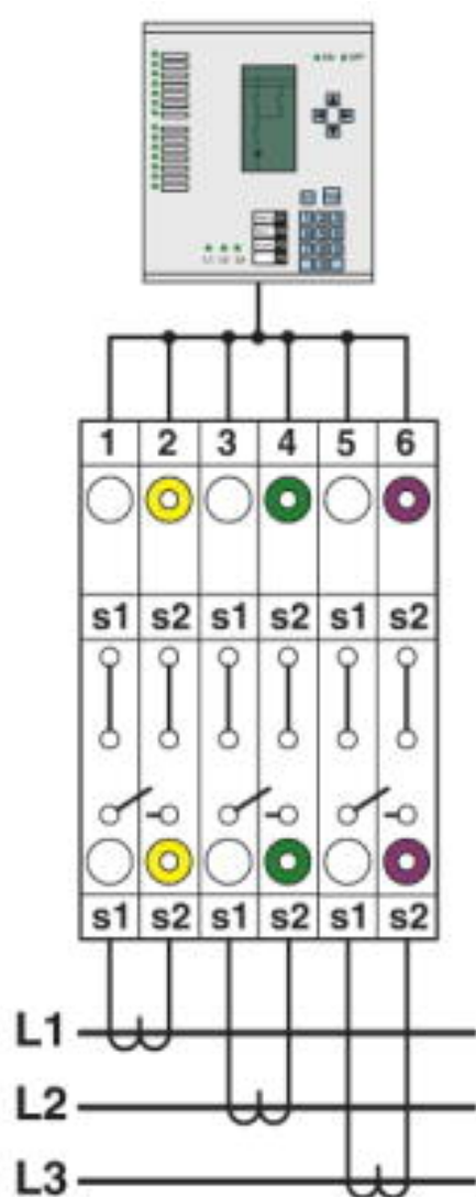
Háromfázisú áramváltókészlet
