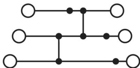
Kapcsolási rajz
