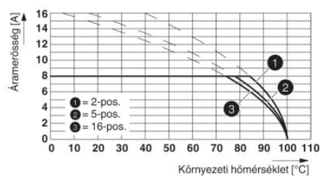
Típus: MC 1,5/...-STF-3,81 DFK-MC 1,5/...-GF-3,81-gyel (forrasztócsatlakozással)
