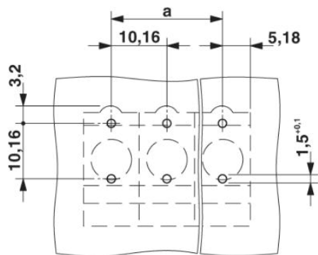
Furatterv/forrasztópád-geometria
