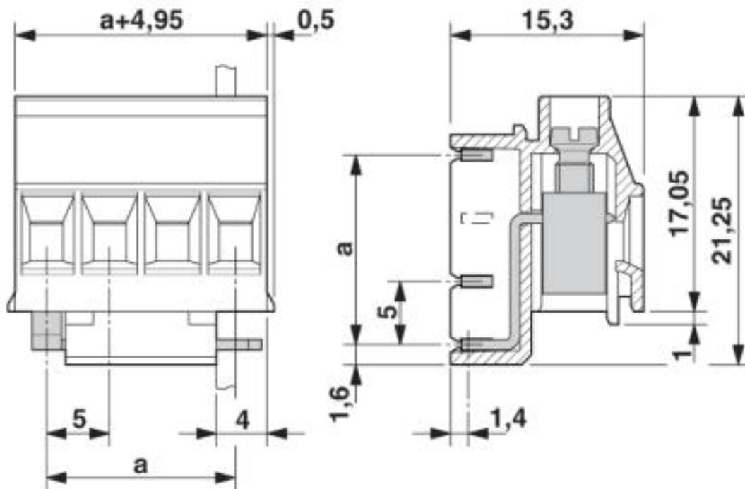
Méretrajz
