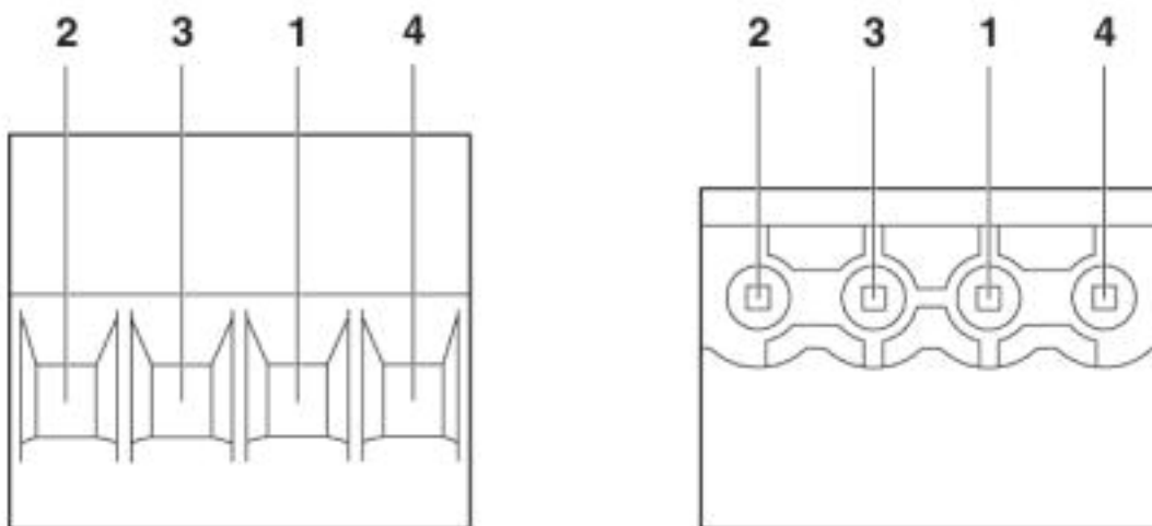
Baloldali lábkiosztás
