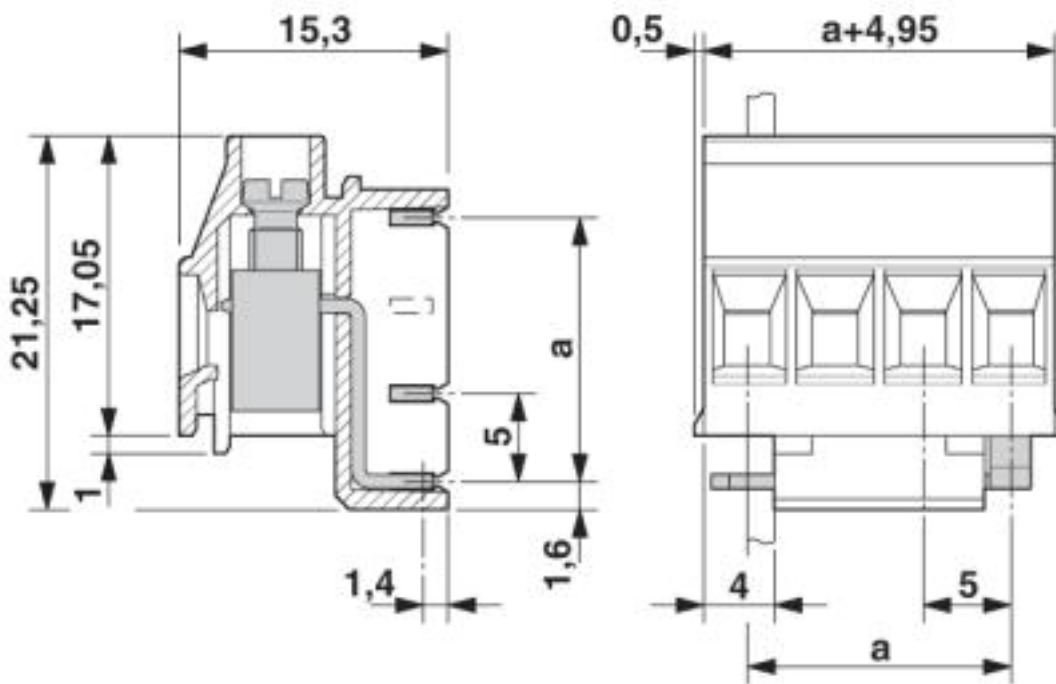
Méretrajz
