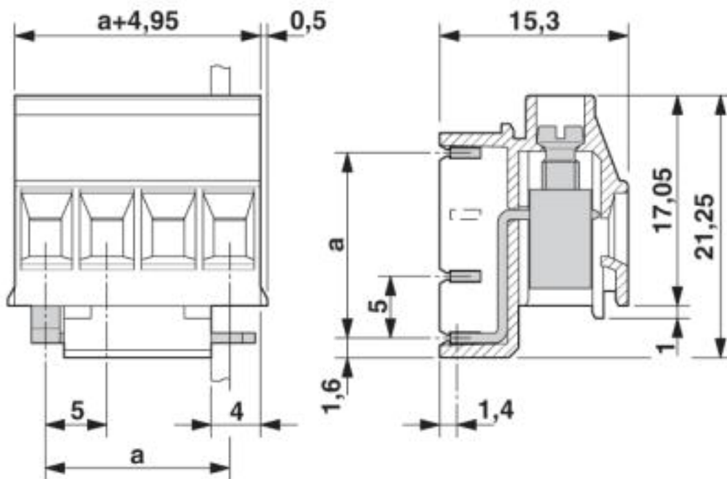
Méretrajz
