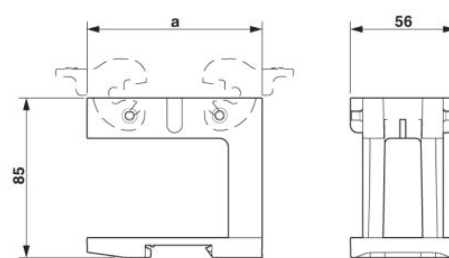
Méreterajz, a = 120
