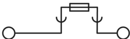
Kapcsolási rajz
