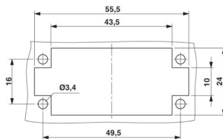
Szerelési kivágás
