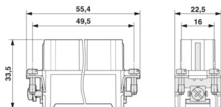
Aljzatbetét
