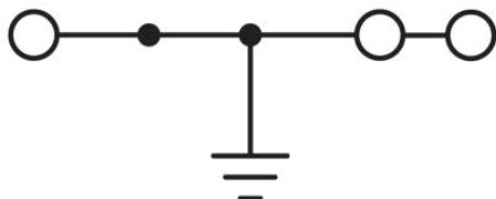
Kapcsolási rajz
