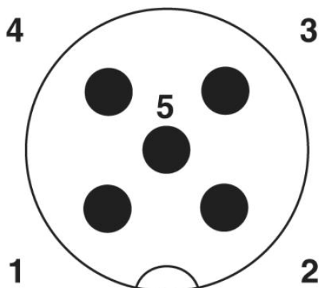
Sematikus rajz
