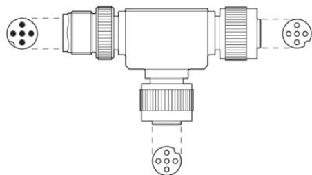
M12 dugasz tűkiosztása, 5 pólusú, "A" kódolás, tűk felől nézve
