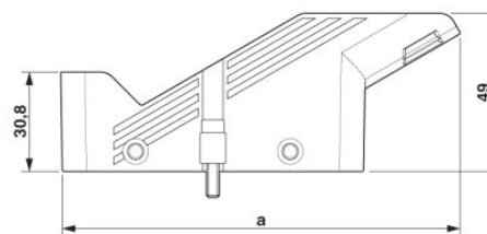
Méreterajz, a = 150,2
