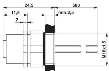
M12 beépíthető aljzat, pozicionálható
