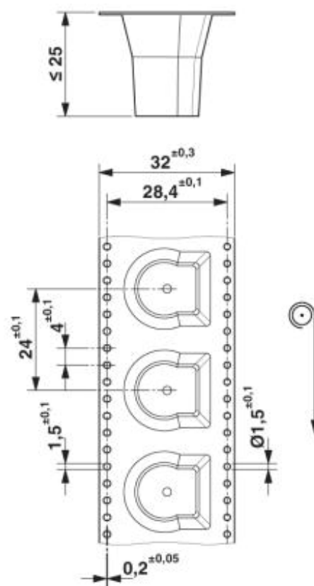
THR hevedercsomagolás (Tape-on-Reel)
