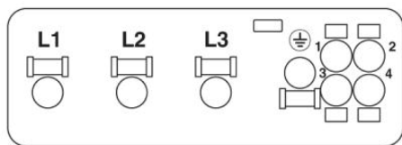
Csatlakozóoldali pólusrajz
