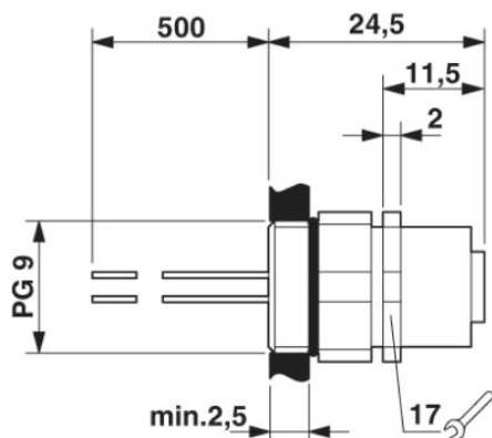
M12 beépíthető dugasz, pozicionálható
