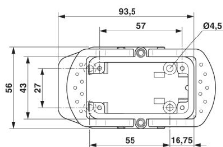
Felülnézeti méreterajz
