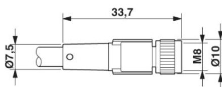
Aljzat M8 x 1, egyenes
