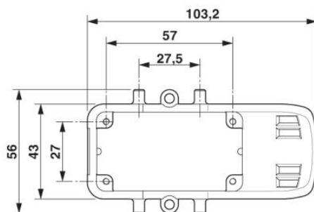
Felülnézeti méretrajz
