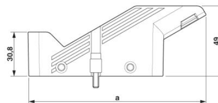
Méretrajz, a = 103,2
