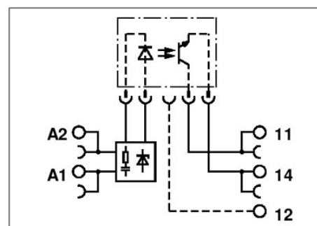
DC kimenet
