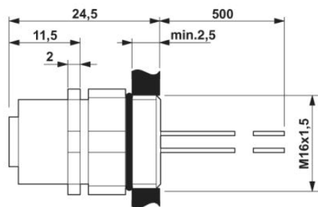
M12 beépíthető aljzat, pozícionálható
