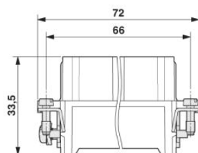
Aljzatbetét
