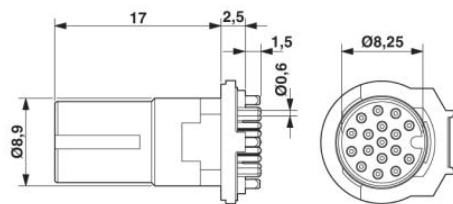
M12 aljzat érintkezőhordozó
