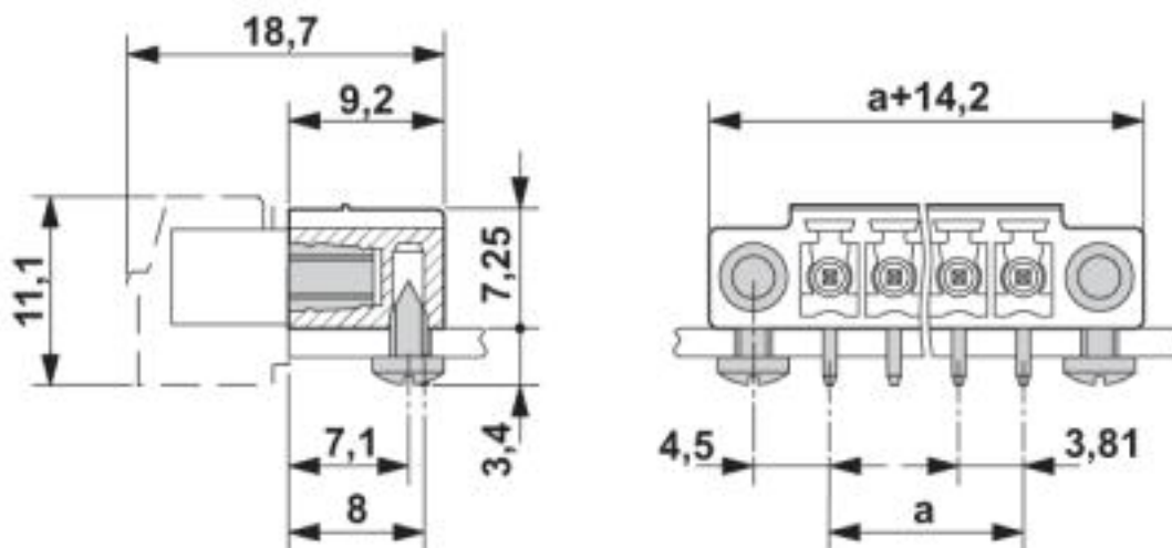
Méretrajz
