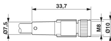
Aljzat M8 x 1, egyenes
