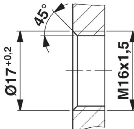
Készülék ház kivágás az M16 rögzítőmenethez, szerelőfal menettel
