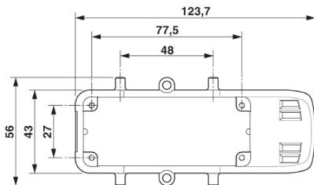
Felülnézeti méreterajz
