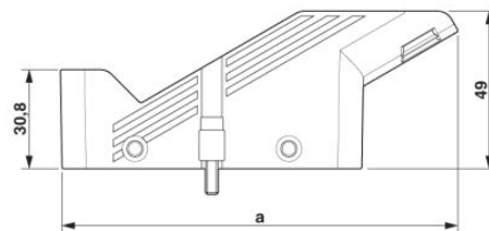
Méreterajz, a = 123,7
