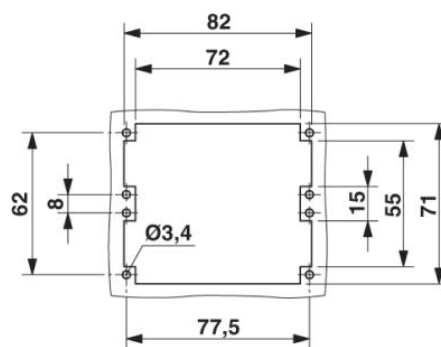
Szerelési kivágás
