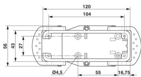
Felülnézeti méretezrajz
