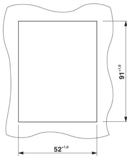
Szerelési kivágás
