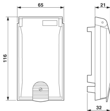
Méretrajz VS-SI-EB-EMV-1
