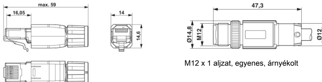
RJ45 csatlakozó, IP20
