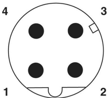
M12 dugasz pólusábrája, 4 pólusú, D kódolású, dugaszoldali nézet
