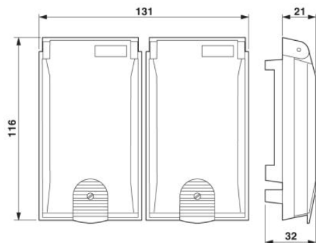
Szerelőkeret
