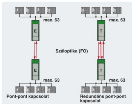
Pont-pont kapcsolat
