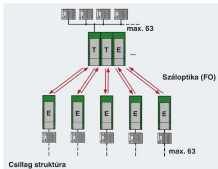
csillag struktúra
